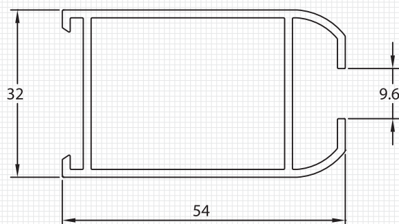
M8811 BASTIDOR MONOLÍTICO Peso : 0.753 Kg./m Espesor : 1.5 mm
