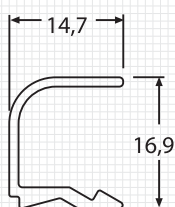
M8803 JUNQUILLO Peso : 0.152 Kg./m Espesor : 1.3 mm
