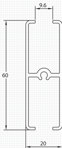
M8816 PALILLO MONOLÍTICO Peso : 0.663 Kg./m Espesor : 1.5 mm
