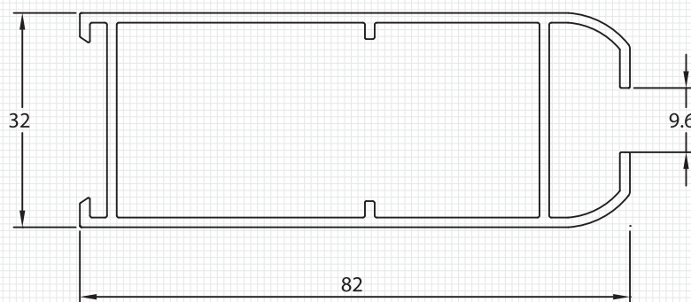
M8815 BASTIDOR MONOLÍTICO Peso : 1.001 Kg./m Espesor : 1.45 mm
