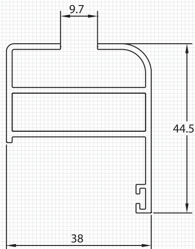
M8832 HOJA MONOLITICO Peso : 0.682 Kg./m Espesor : 1.5 mm
