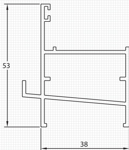
M8835 CAMARA DE CONDENSACION Peso : 0.751 Kg./m Espesor : 1.5 mm
