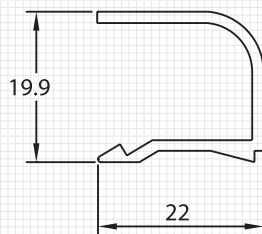
M8833 JUNQUILLO MONOLITICO Peso : 0.245 Kg./m Espesor : 1.5 mm
