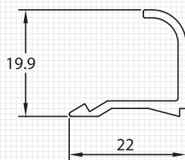
M8837 JUNQUILLO TP Peso : 0.192 Kg./m Espesor : 1.5 mm
