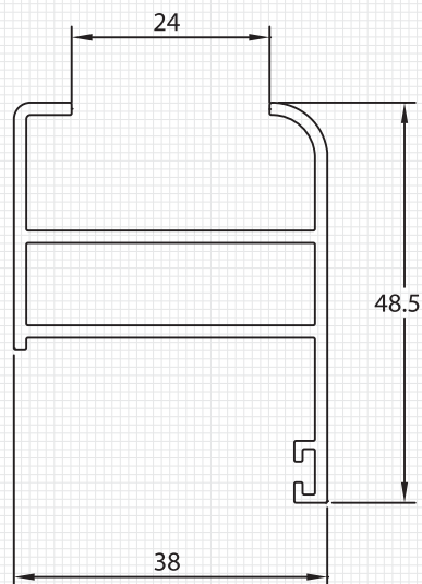
M8836 HOJA TP Peso : 0.660 Kg./m Espesor : 1.5 mm
