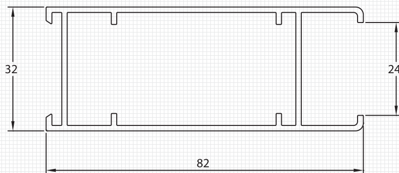
M8817 BASTIDOR TP Peso : 0.999 Kg./m Espesor : 1.4 mm
