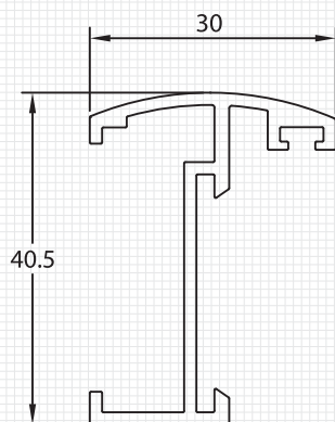
M8812 MARCO Peso : 0.467 Kg./m Espesor : 1.5 mm
