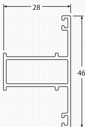
M8804 PALILLO Peso : 0.415 Kg./m Espesor : 1.3 mm
