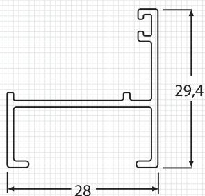
M8801 MARCO Peso : 0.265 Kg./m Espesor : 1.3 mm
