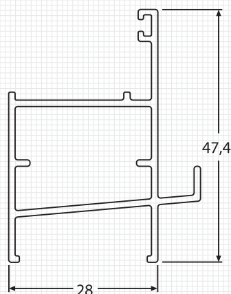
M8805 CAMARA DE CONDENSACIÓN Peso : 0.516 Kg./m Espesor : 1.3 mm
