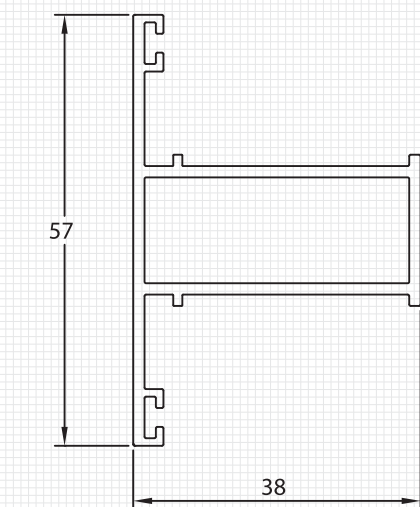
M8834 TRAVESANO Peso : 0.650 Kg./m Espesor : 1.5 mm
